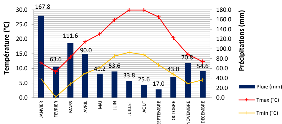
Diagramme ombrothermique 2018
